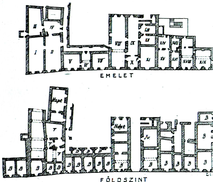
AZ 1839-BEN ELBONTOTT RÉGI VÁROSHÁZA ALAPRAJZA.
