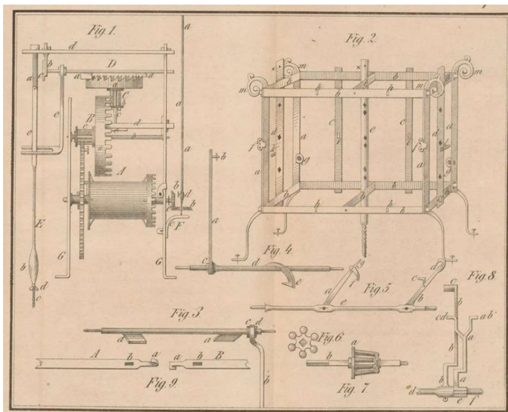
11. kép. Egy 1846-ban megjelent, a toronyórák készítésével és javításával foglalkozó szakkönyv egyik mellékletén (a műszaki rajz bal oldalán) ingaszabályozós, orsógátlású óraszerkezet látható.
