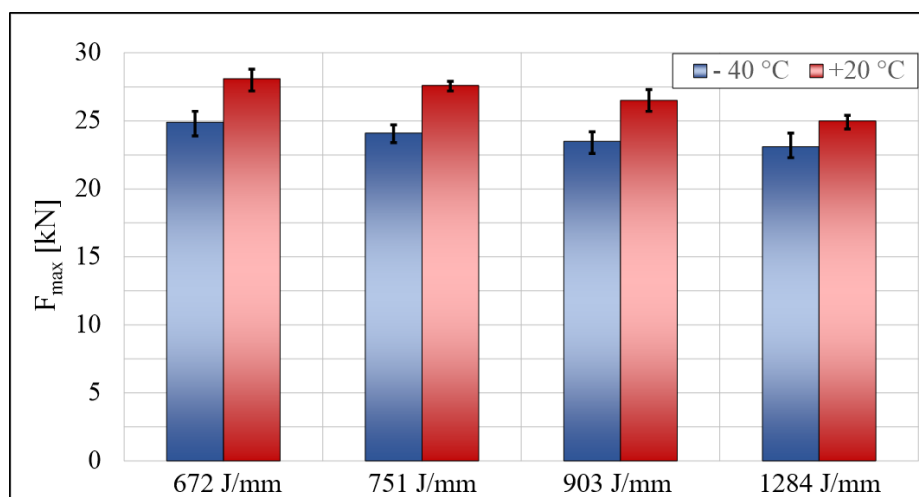
5. ábra: A maximális üttöerő értékek különböző hőbevitelnél, mindkét hőmérsékleten
