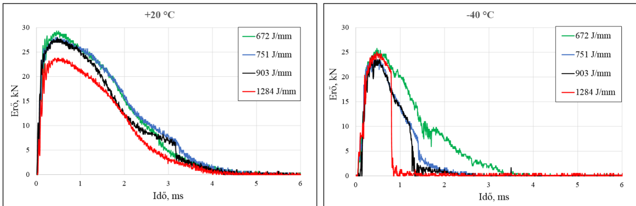
6. ábra: Az ütővizsgálat erő – idő görbéi +20 °C és -40°C-on
