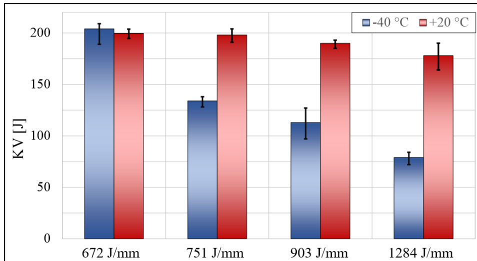
4. ábra: Az ütmunka értékek különböző hőbevitelnél, mindkét hőmérsékleten
